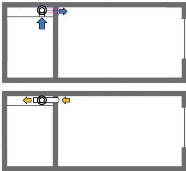
Abbildung 4.3 Variante mit aktiven Überströmern, die Luft in die Abhangdecke rückführen (Quelle: Rojas-Kopeinig, G.)
