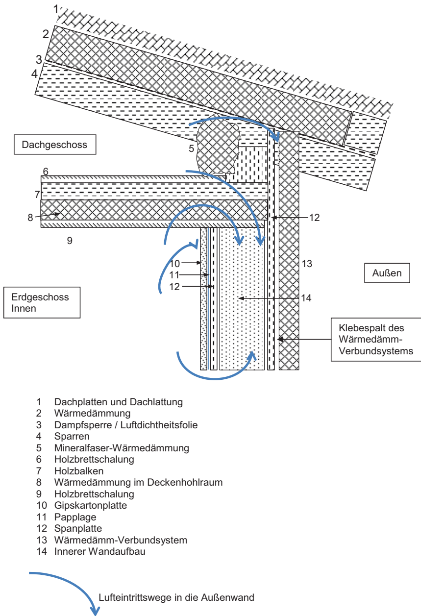
Abb. 10.23: Lufttrittswege in die Holzständer-Außenwand (schematische Skizze, ohne Maßstab)
