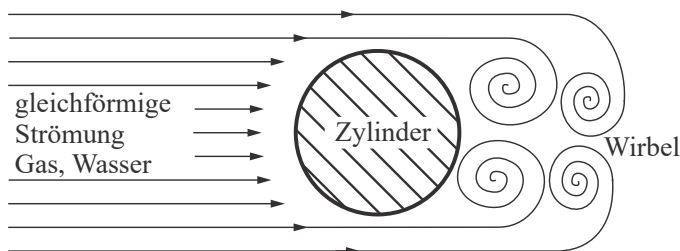
Abb. 1.4: Karman'sche Wirbelbildung als Querschwingung am Turmbauwerk
